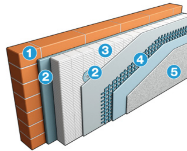
Aufbauschema Wärmedämm-Verbundsystem
